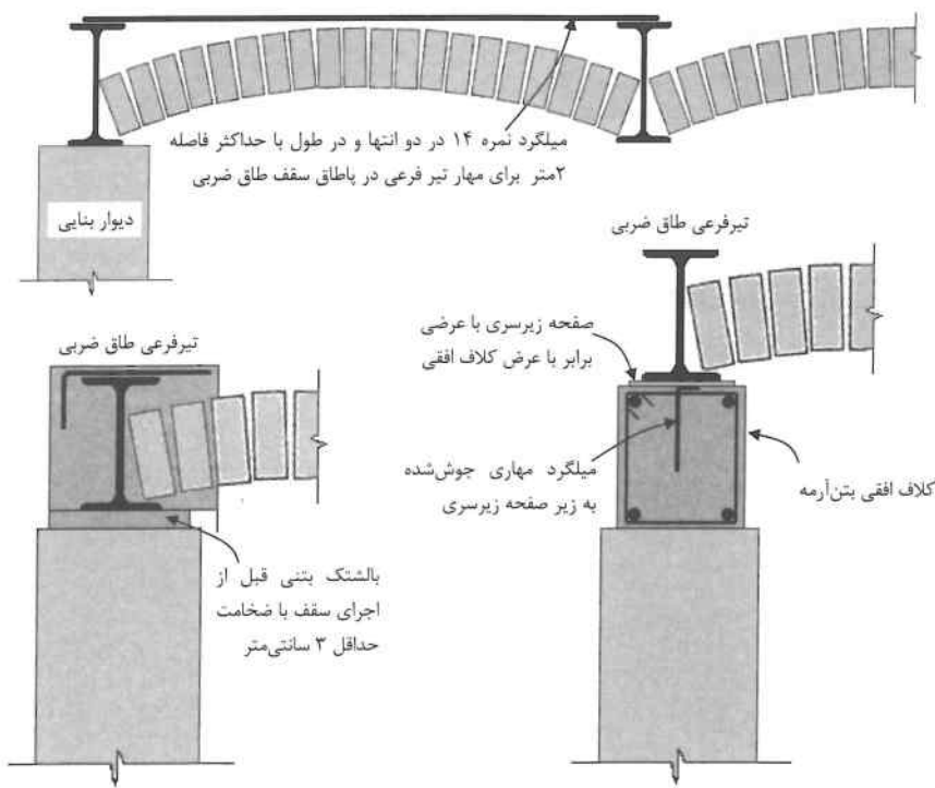
ب- ترکیب تیرفرعی باطاق یا کلاف افقی
