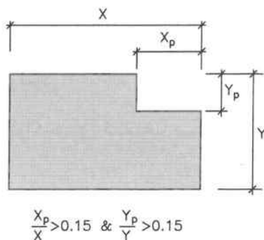
الف - نامنظمی هندسی
