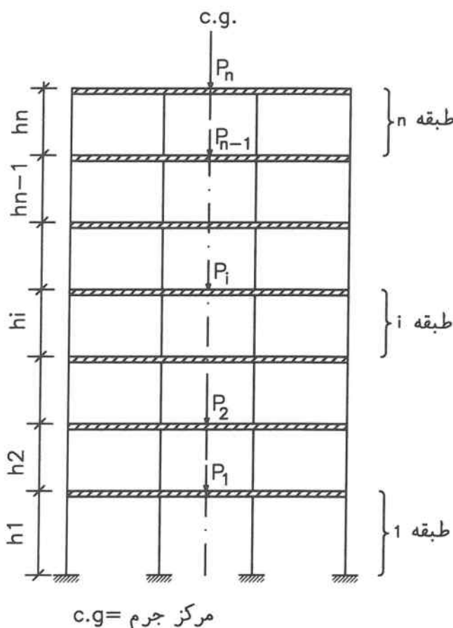
شکل پ-۳-۱ سازه چند طبقه تحت اثر بارهای قائم
