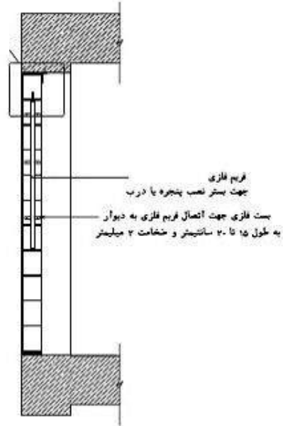
بشرش A-A
