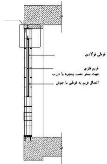
بشرش A-A
